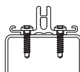
Sur profilé creux épaisseur mini. 2 mm
