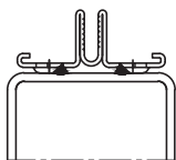
Sur profilé creux épaisseur mini. 3 mm
